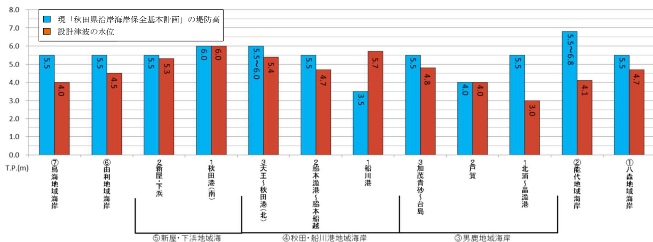
【設計津波の水位】
