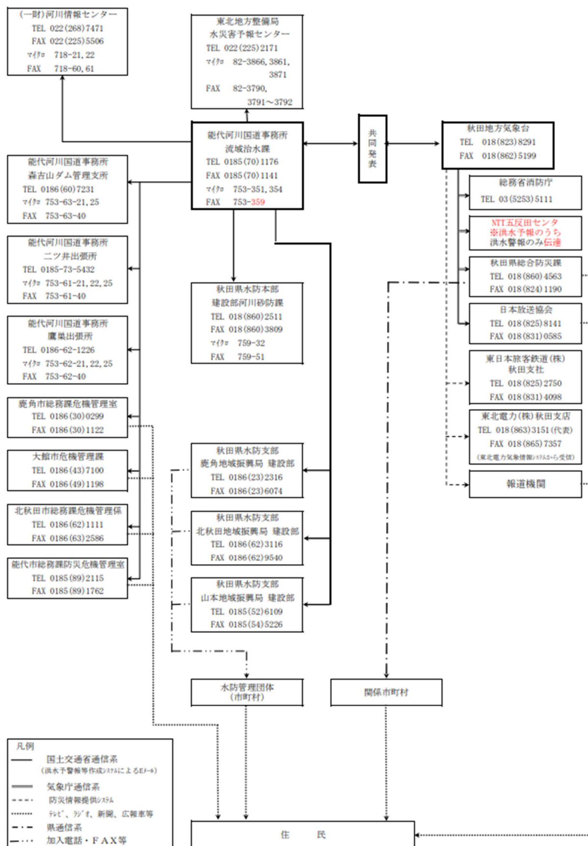
【米代川（藤子川を含む）の指定河川洪水予報伝達系統図（大臣・気象庁長官共同発表）】
