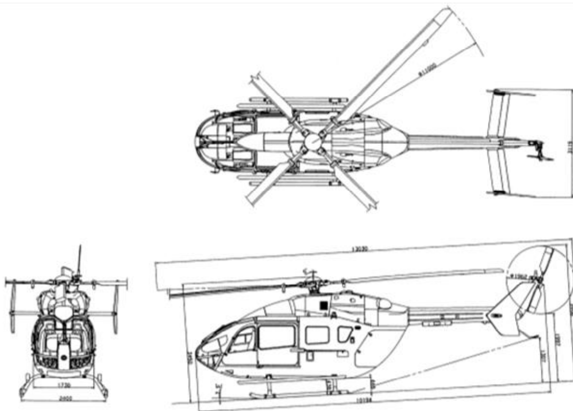
三面図 ー BK117C-2 型
